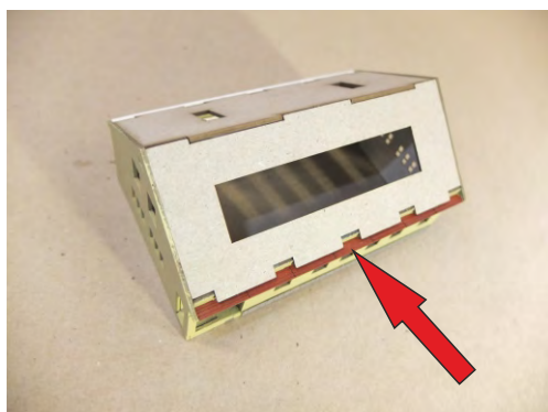
Nalepení nabarvené ho spodního podbití a vlepění střešních výstuh.
